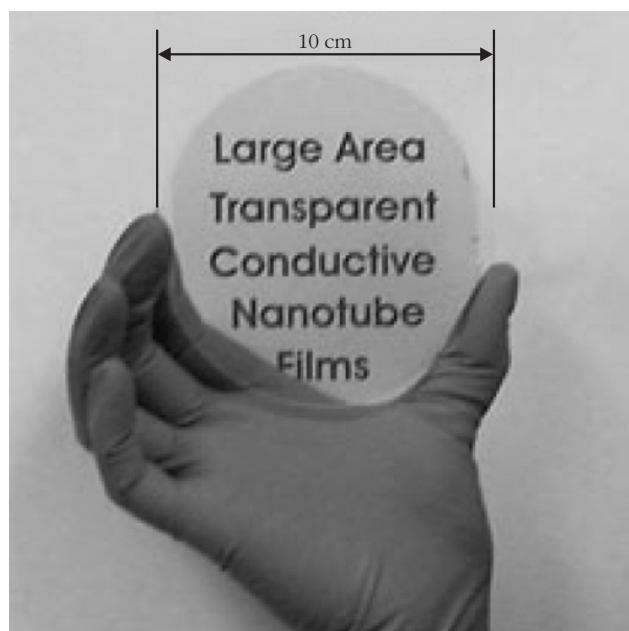
6. ábra. 80 nm vastagságú, egyfálú szén nanocsövekből álló film, zafír hordozón. Az olvasható szöveg a film mögött van. ( Science 305 (2004) 1273)
