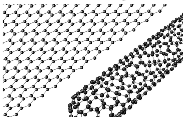
1. ábra. Szén nanocső származtatása hatszöges rács feltekeréséből
